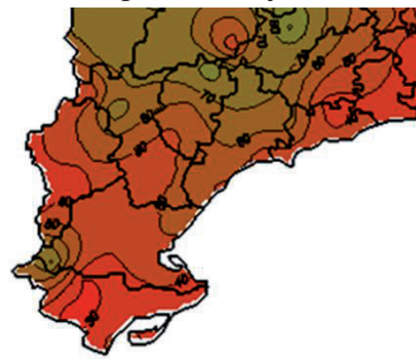
% Pluviometria a 3 mesos gener – març 16
