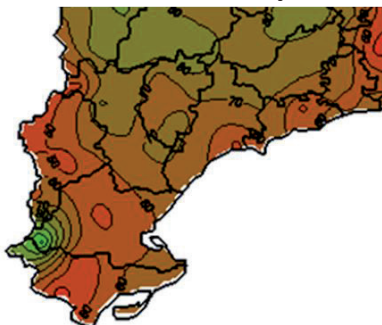
% Pluviometria a 6 mesos octubre 15 – març 16
