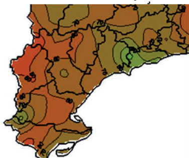
% Pluviometria a 12 mesos abril 15 – març 16
